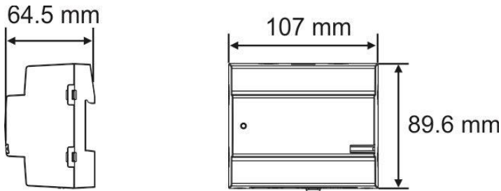
尺寸图
