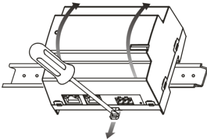
拆卸图
