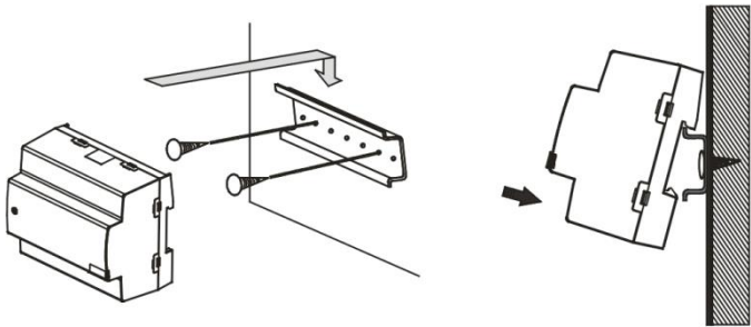
安装图
